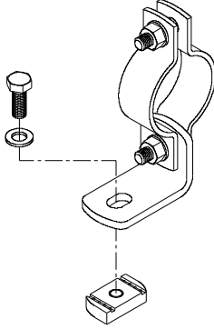
batten clip & angle bracket 18-00-36
